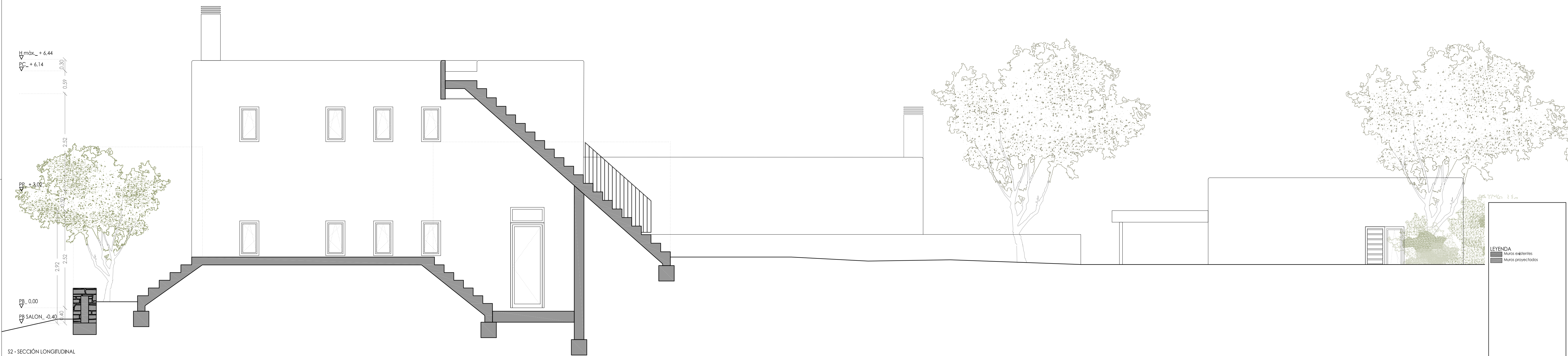
S2 - SECCIÓN LONGITUDINAL
