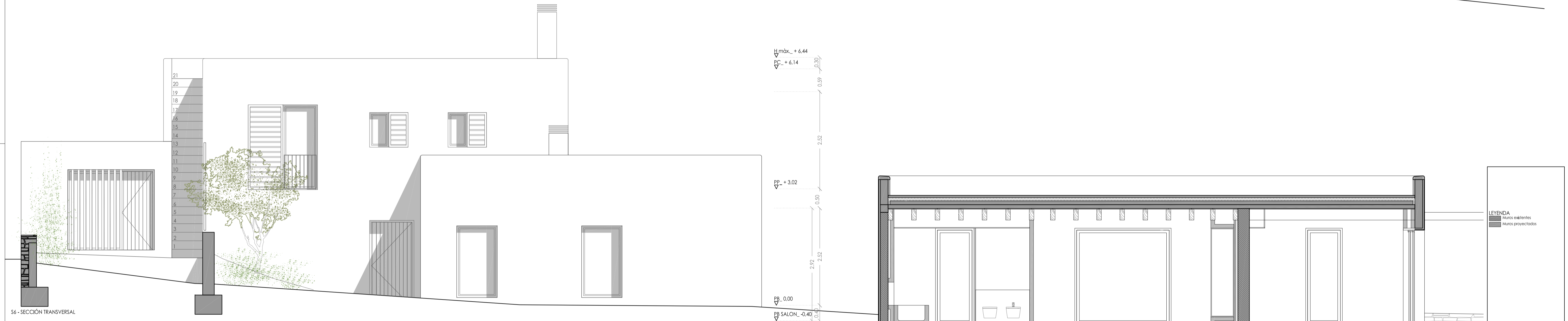
FACHADA OESTE
