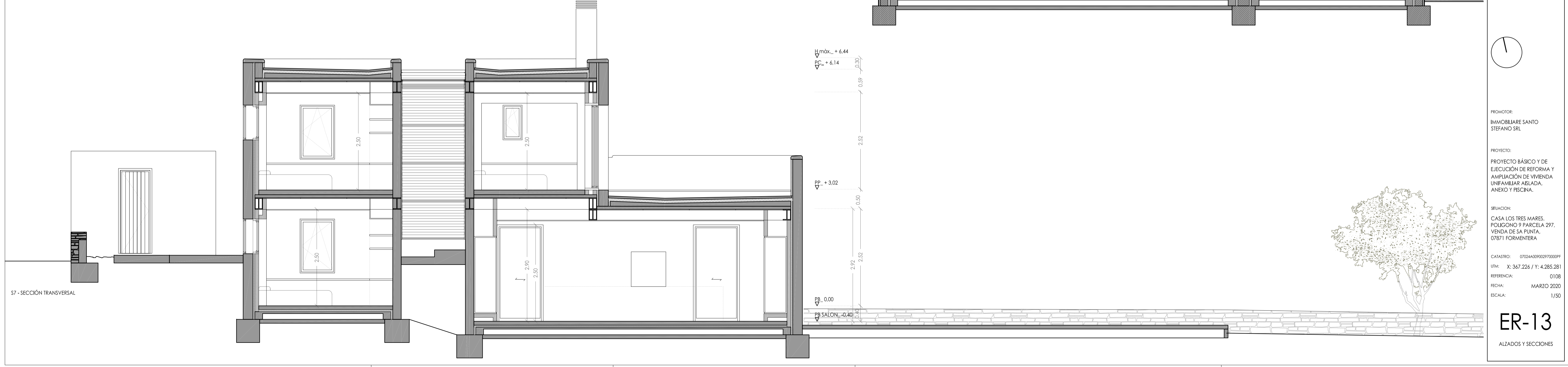
S6 - SECCIÓN TRANSVERSAL
